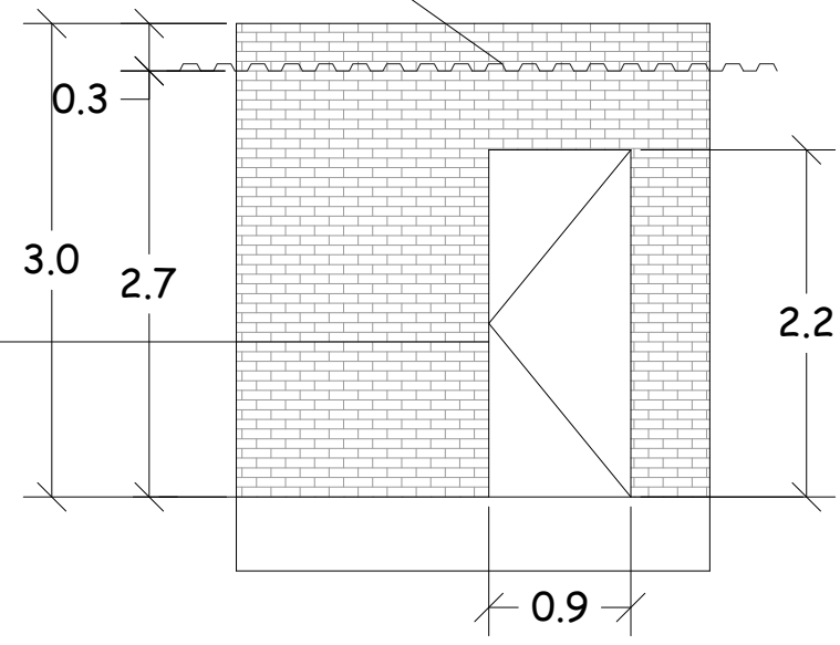
4 SECTION A-A
